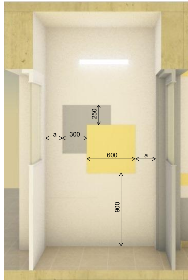
Розгортка 3-4
